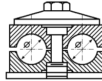
Collare Polipropilene Tipo CF
